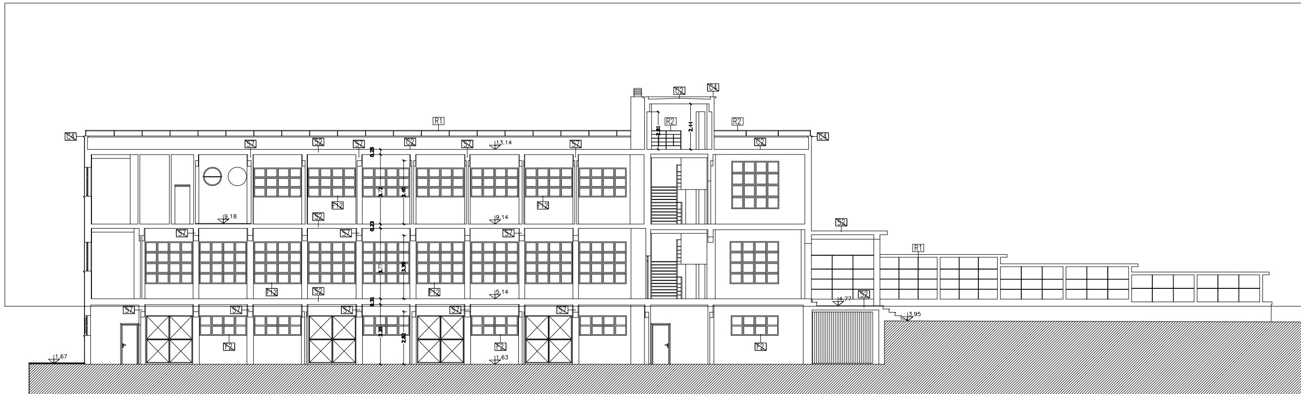
SEZIONE "C-C"
