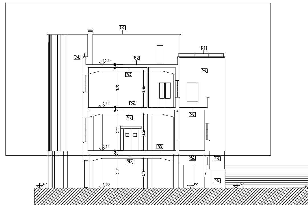
SEZIONE "E-E"
